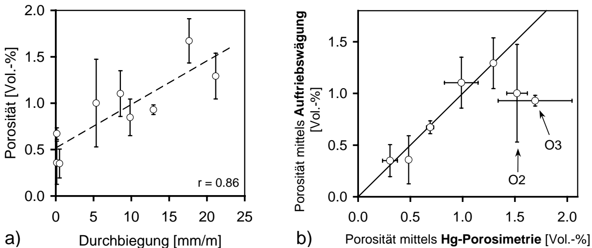
Abb. 8.9: Nutzporosität der demontierten Marmorplatten. a) Porosität aus der Auftriebswägung als Funktion der Durchbiegung. Eingetragen sind die Regressionsgerade (gestrichelte Linie) und der Korrelationskoeffizient ( r ). b) Vergleich der Porositätswerte aus zwei Verfahren. Die durchgezogene Linie markiert identische Werte. Die Fehlerindikatoren markieren die Standardabweichung.
