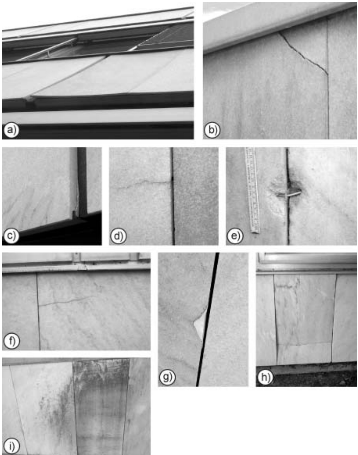
Abb. 4.5: Schadensphänomene an der Fassadenverkleidung der drei untersuchten Gebäude. a) Konkave Einschüselung. b) Durchgehender Riss an der oberen Plattenecke, der sich leicht zum Ausbruch entwickelt. c) Riss, initiiert an der unteren Nut. d) Riss, initiiert am Ankerdorn. e) Durch die Plattenverformung verbogener Ankerdorn (rechts), sichtbar durch die Abplatzung am Halteanker. f) Langer Riss verläuft quer durchs Platteninnere. g) Mit Ersatzmasse verspachtelter Ausbruch (Juridicum). h) Gebrochene Marmorplatte in der untersten Fassadenzeile als Folge von Vandalismus. i) Mit Biofilm besiedelte Fassadenplatte (rechts).
