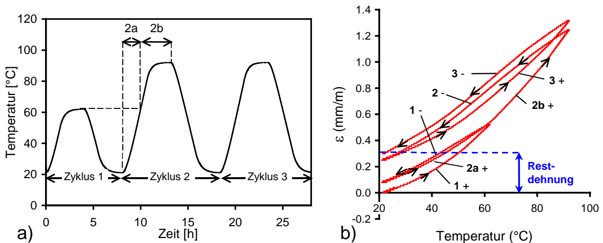
Abb. 3.3: a) Temperaturverlauf während der Dilatationsmessung beim Durchlaufen der drei Heizzyklen. Die Heiz- und Abkühlrate beträgt 0,5\text{ °C}/\text{min} . Die Maximaltemperatur in Zyklus 1 ist 60\text{ °C} , in Zyklus 2 und 3 jeweils 90\text{ °C} . b) Beispiel einer Dehnungskurve beim Durchlaufen der drei Heizzyklen. +: Heizphase; -: Abkühlphase.
