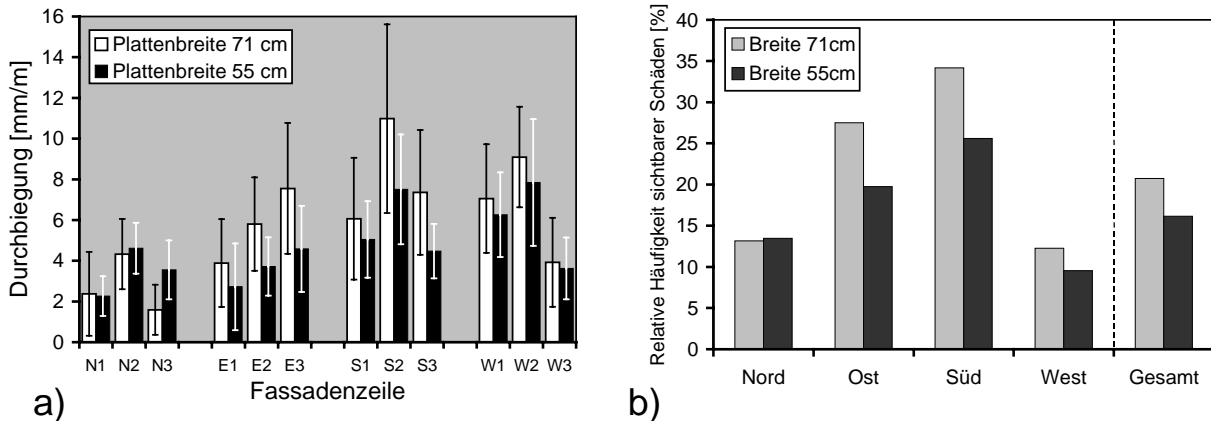
Abb. 4.10: Zusammenhang zwischen Plattenbreite und Schädigungsgrad an den Marmorplatten des Juridicums: a) Zeilenmittelwerte der Durchbiegung in Abhängigkeit der Plattenbreite (die Fehlerindikatoren markieren die Standardabweichung); b) Relative Schadenshäufigkeiten der Fassadenplatten in Abhängigkeit der Plattenbreite.
