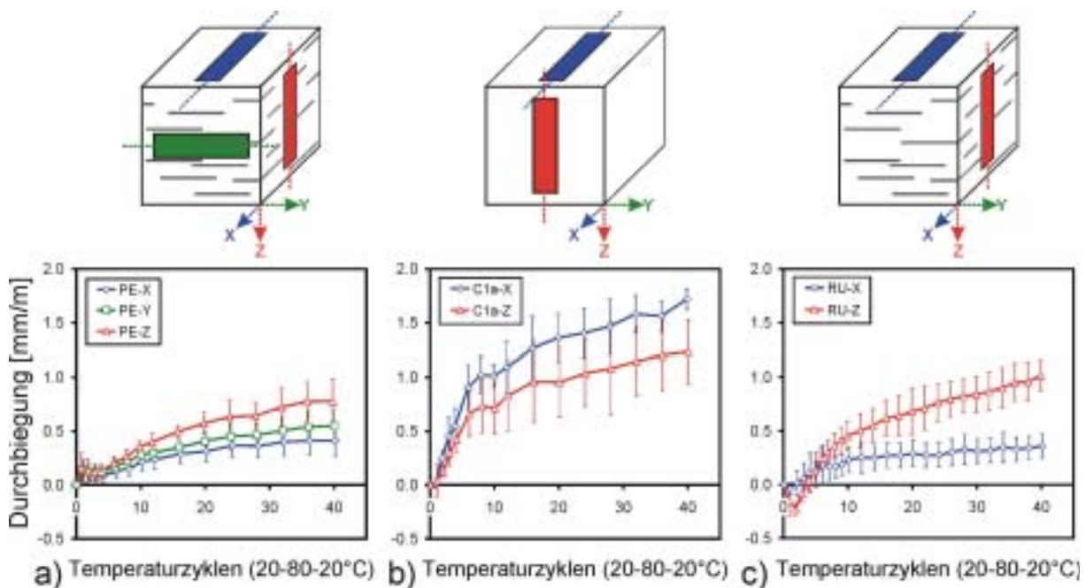
Abb. 6.12: Durchbiegung von Marmorplatten als Funktion der Anzahl von Temperaturzyklen der Marmore a) Peccia, b) Carrara 1a und c) Ruivina (aus Koch & Siegesmund 2004b). Die Kurven geben den mittleren Verlauf von jeweils drei Probekörper der gleichen Schnittlage wieder. Die Fehlerindikatoren markieren die Standardabweichung. Die Würfel stellen schematisch die Orientierung der Probekörper dar, deren Farbe mit den Kurven korrespondiert.
