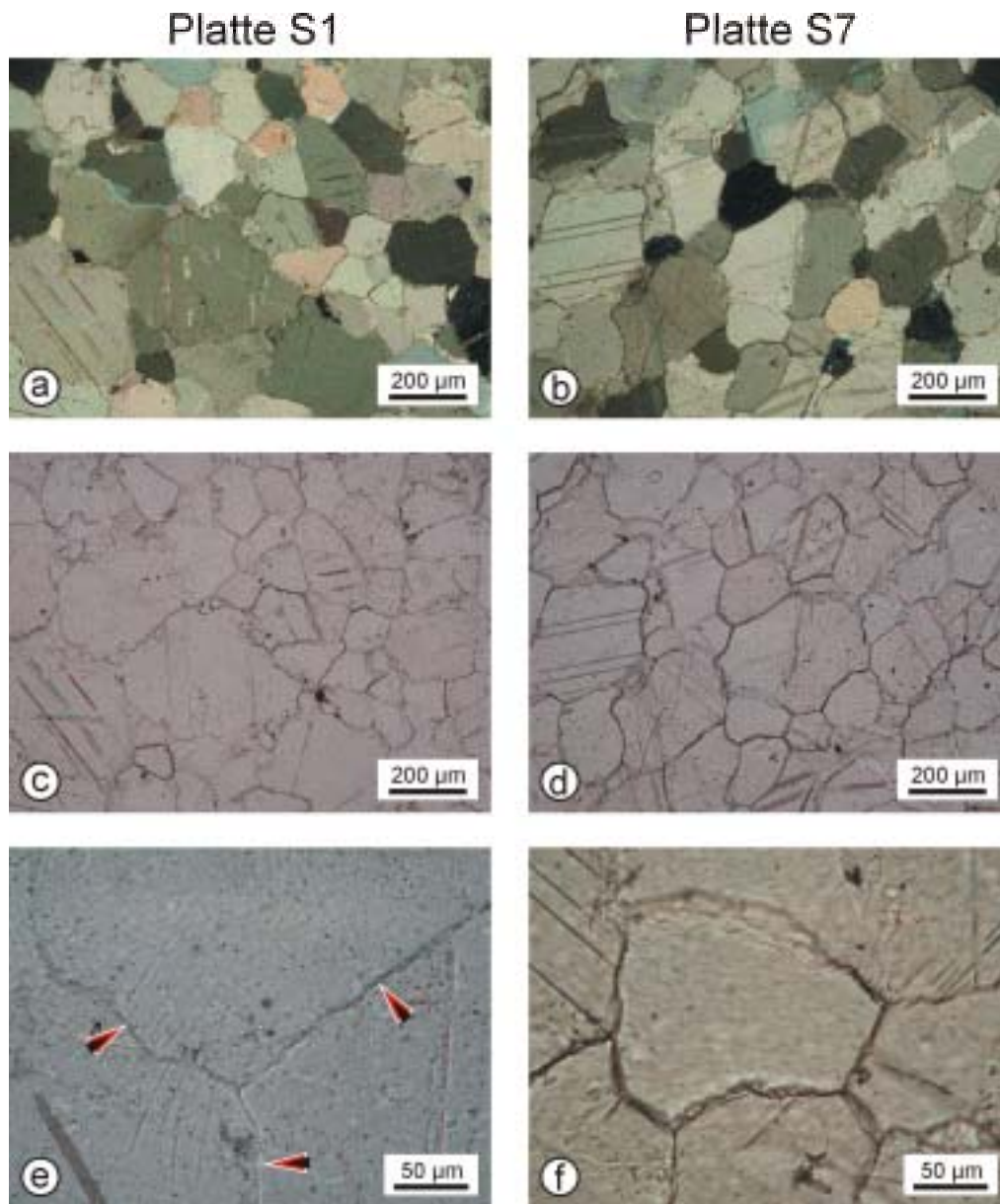
Abb. 8.20: Mikrogefüge der schwach verformten Platte S1 (linke Seite) und der stark verformten Platte S7 (rechte Seite). a,b Übersicht (gekreuzte Polarisatoren). c,d Jeweils gleicher Bildausschnitt wie im Bild darüber (Durchlicht). e,f Detailaufnahme der Korngrenzen (Durchlicht). Die Korngrenzen des Marmors der Platte S7 sind deutlich stärker geöffnet als die der Platte S1 (Pfeile).
