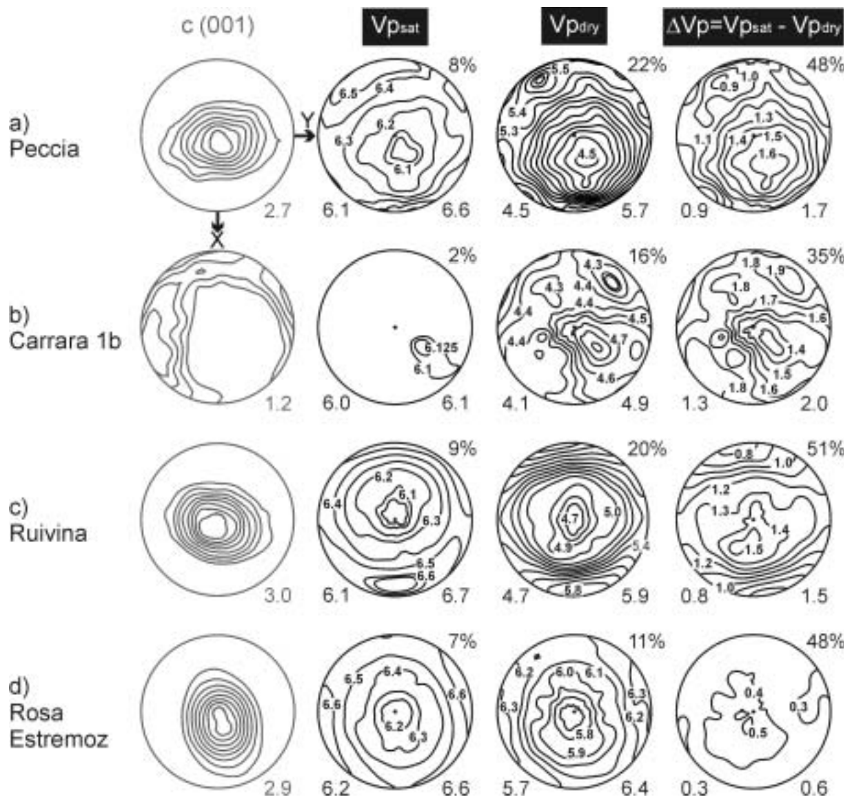
Abb. 5.26: V_P -Verteilung von Kugelproben im wassergesättigten ( V_{P,sat} ) und im trockenen ( V_{P,dry} ) Zustand sowie die Geschwindigkeitsdifferenzen aus beiden Zuständen ( \Delta V_P ; untere Halbkugel; stereographische Projektion). Die Polfiguren der c-Achsen sind jeweils vergleichend dargestellt. Die Isolinien repräsentieren km/s (mit Zahlenangaben) bzw. Vielfache der Gleichverteilung. Die Orientierung ist in der Polfigur links oben markiert. Die Z-Richtung steht senkrecht zur Papierebene. Die Zahlen unter den einzelnen V_P -Polfiguren kennzeichnen die Extrema der Kompressionswellengeschwindigkeit in km/s. Die Prozentwerte geben die Anisotropie von V_P bzw. \Delta V_P an.
