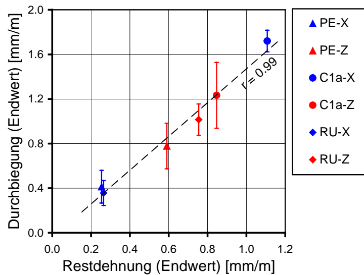
Abb. 6.13: Zusammenhang zwischen thermo-hygrisch induzierter Restdehnung und Plattenverbiegung. Es sind die Endwerte aus Abb. 6.10 und Abb. 6.12 miteinander korreliert. Die Regressionsgerade (gestrichelte Linie) und der Korrelationskoeffizient ( r ) sind gegeben.
