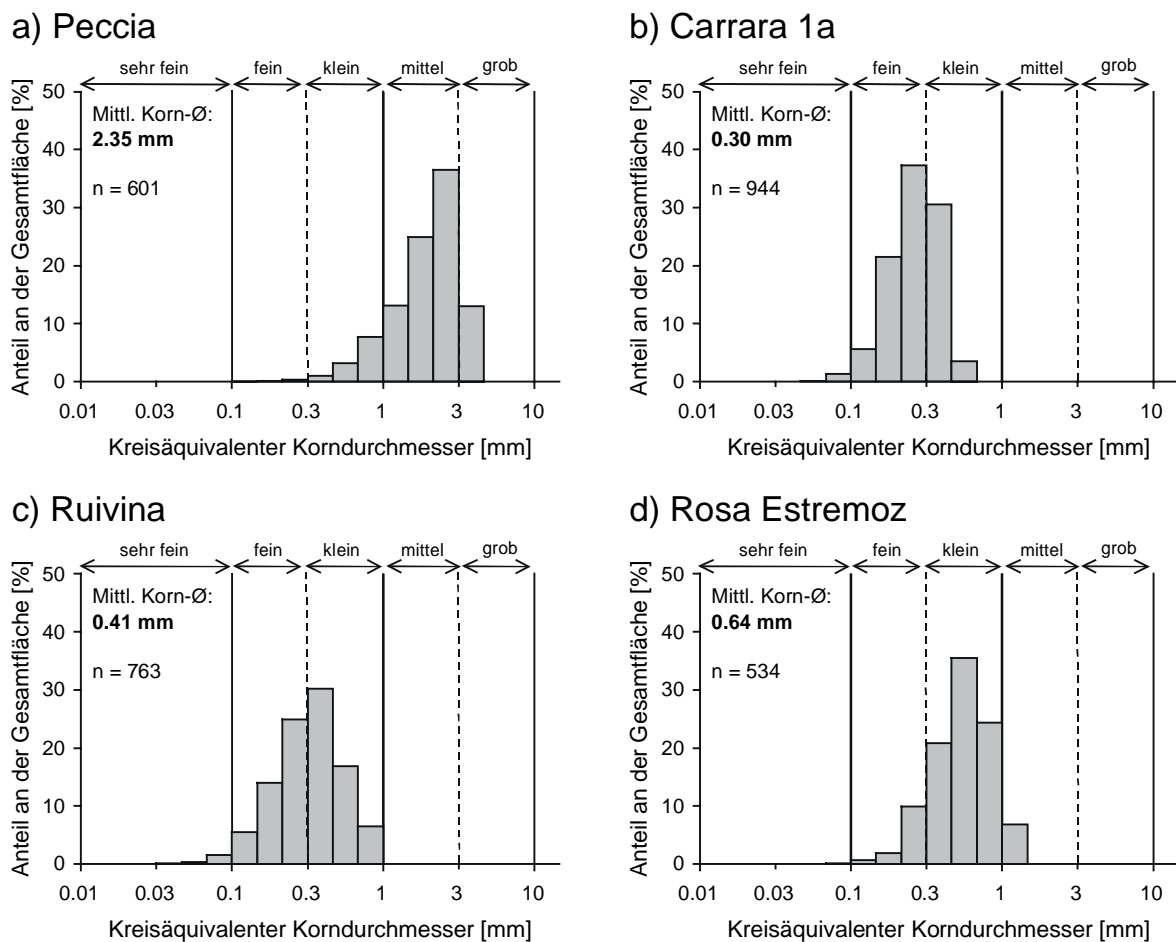
Abb. 5.23: Korngrößenverteilung der Marmore a) Peccia, b) Carrara 1a, c) Ruivina und d) Rosa Estremoz. Die Korndurchmesser sind im logarithmischen Maßstab aufgetragen. Die Korngrößenbezeichnung „sehr fein“ bis „grob“ erfolgte nach Wimmenauer 1985 (vgl. Tab. 2.1).
