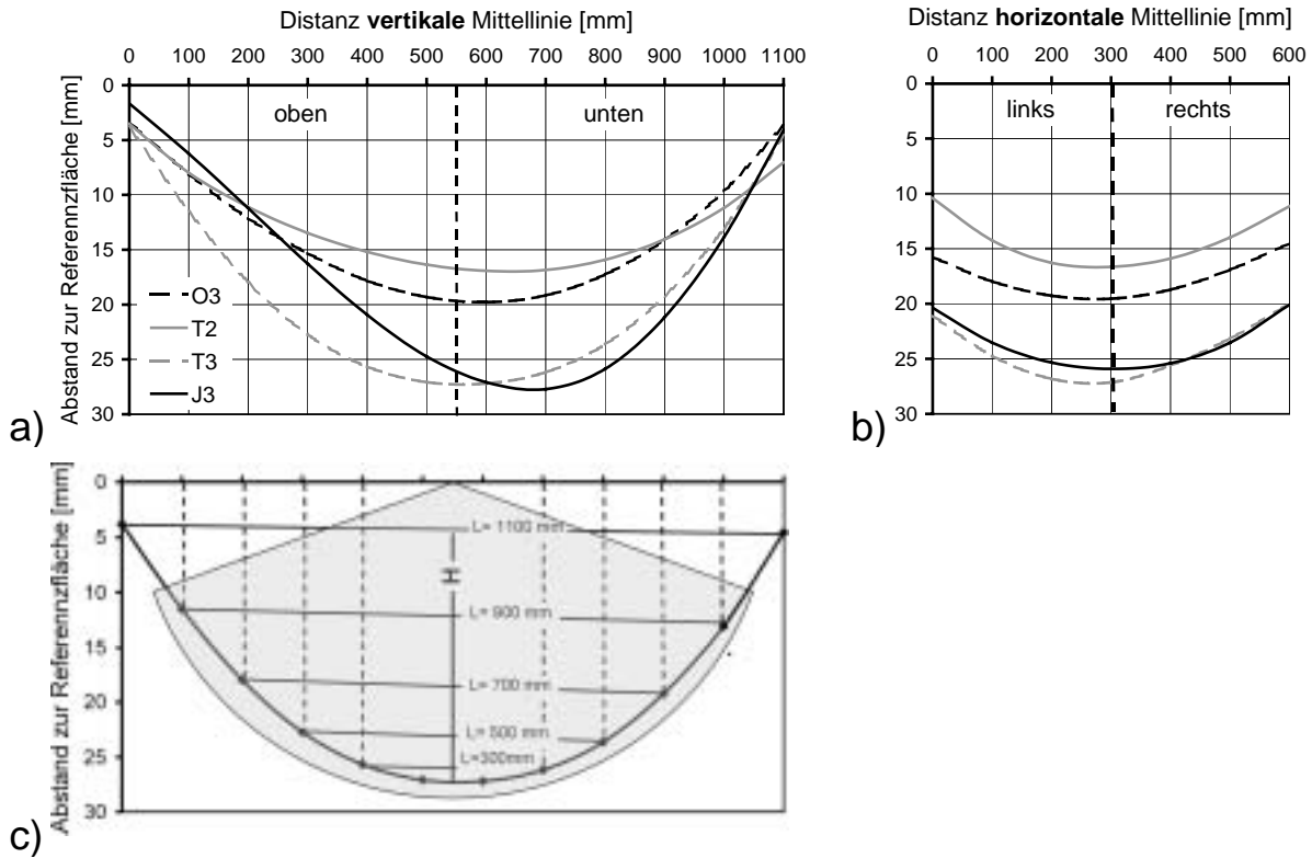
Abb. 8.3: Überhöhte Querprofile durch verbogene Fassadenplatten: a) Längsschnitte durch die vertikale Mittellinie; b) Querschnitte durch die horizontale Mittellinie; c) Vergleich zwischen der Krümmung einer Fassadenplatte und der eines Kreissegmentes am Beispiel des Längsschnittes durch die vertikale Mittellinie der Platte T3. Die Berechnung der Durchbiegungen B über verschiedene Messabstände L hinweg sollte zu vergleichbaren Ergebnissen führen.
