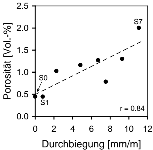
Abb. 8.21: Zusammenhang zwischen Porosität und Plattenverbiegung am Beispiel der acht demontierten Fassadenplatten: Eine Innenplatte (S0) und sieben Außenplatten (S1 bis S7). Eingezeichnet sind die Regressionsgerade (gestrichelte Linie) und der Korrelationskoeffizient ( r ).
