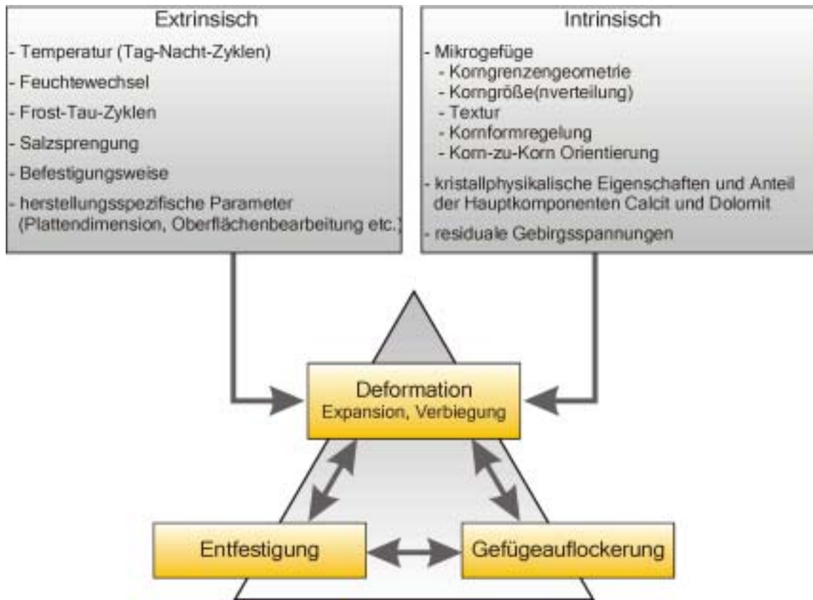
Abb. 2.9: Grundschema des Zusammenwirkens von Einflussparametern auf die Verwitterung von Marmorplatten.
