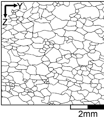
Abb. 5.21: Korngefüge in jeweils drei orthogonalen Schnitlagen der Marmore a) Peccia, b) Carrara 1a, c) Ruivina und d) Rosa Estremoz.
