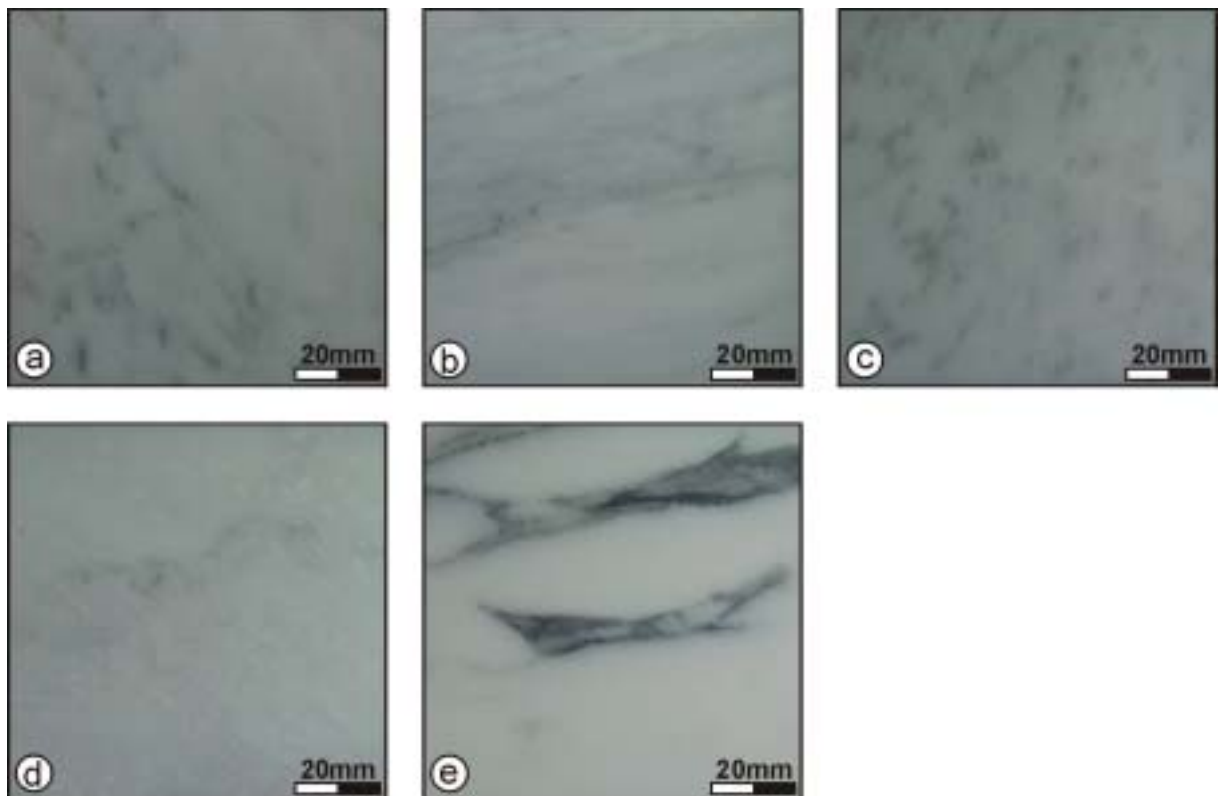
Abb. 5.7: Makroskopisches Erscheinungsbild unterschiedlicher Varietäten des Carrara Marmors: a) Carrara 2 (Arabescato Cervaiole), b) Carrara 3 (Bianco Tre Fiumi), c) Carrara 4 (Canaloni), d) Carrara 5 (Bianco Buca), e) Carrara 6 (Arabescato Corchia).
