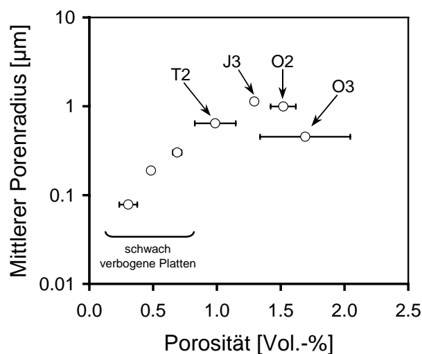
Abb. 8.11: Mittlerer Porenradius als Funktion der Porosität aus der Hg-Porosimetrie. Die Fehlerindikatoren markieren die Standardabweichung.
