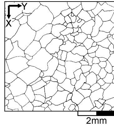
Abb. 5.21: Korngefüge in jeweils drei orthogonalen Schnitlagen der Marmore a) Peccia, b) Carrara 1a, c) Ruivina und d) Rosa Estremoz.
