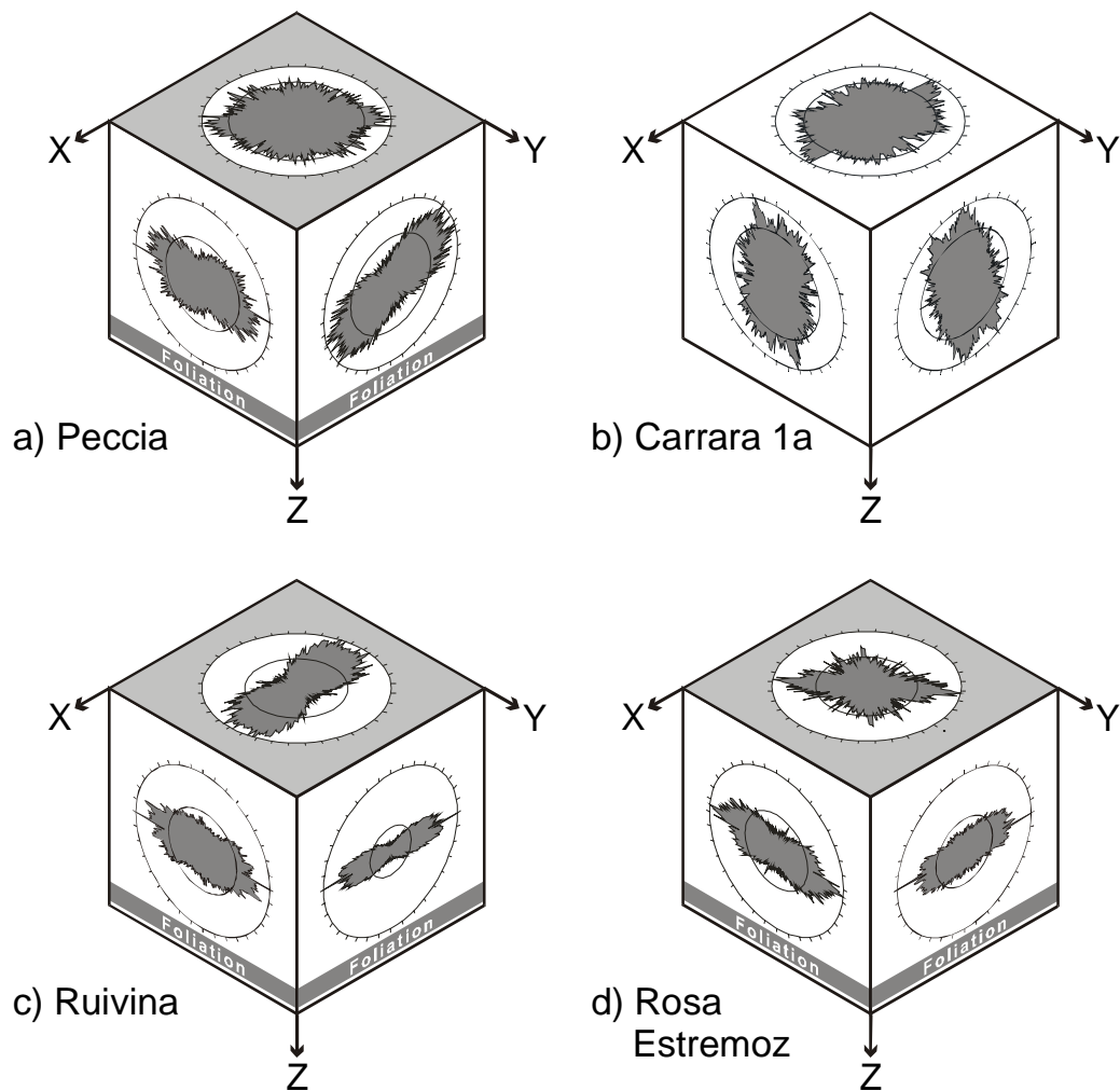
Abb. 5.22: Statistische Verteilung der Korngrenzenorientierung in jeweils drei orthogonalen Schnittlagen der Marmore a) Peccia, b) Carrara 1a, c) Ruivina und d) Rosa Estremoz. Die Innenkreise markieren die Gleichverteilung.
