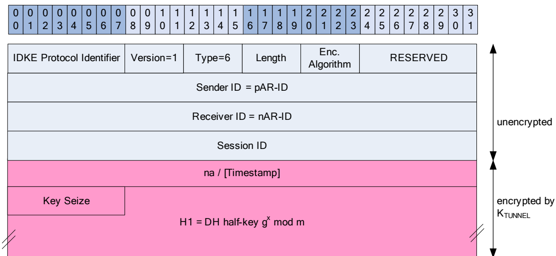
IDKE Message No. 6
