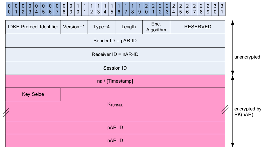
IDKE Message No. 4
