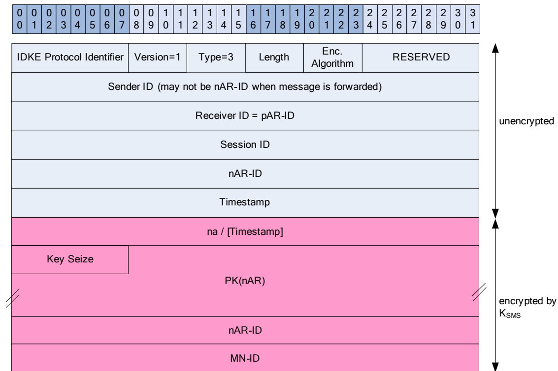
IDKE Message No. 3
