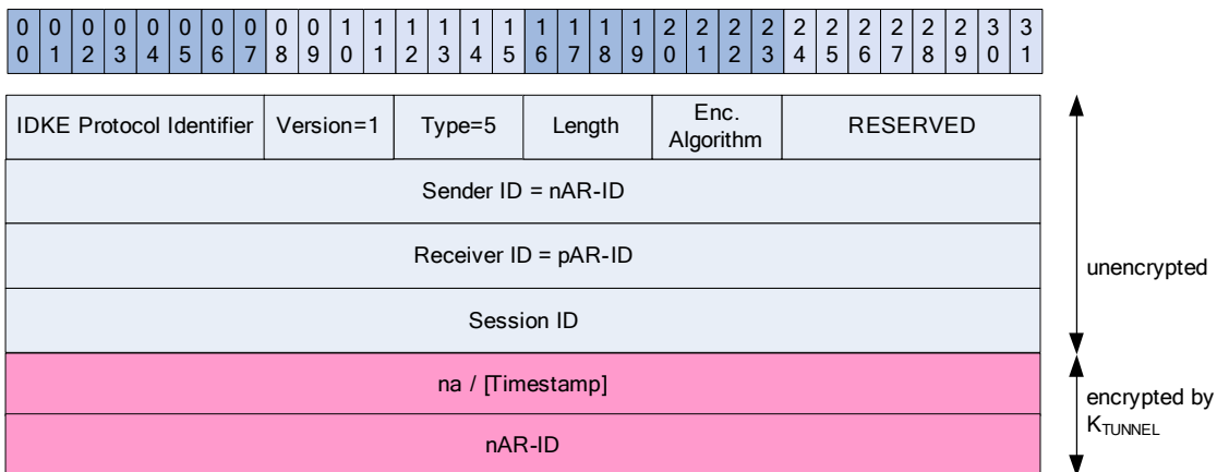
IDKE Message No. 5
