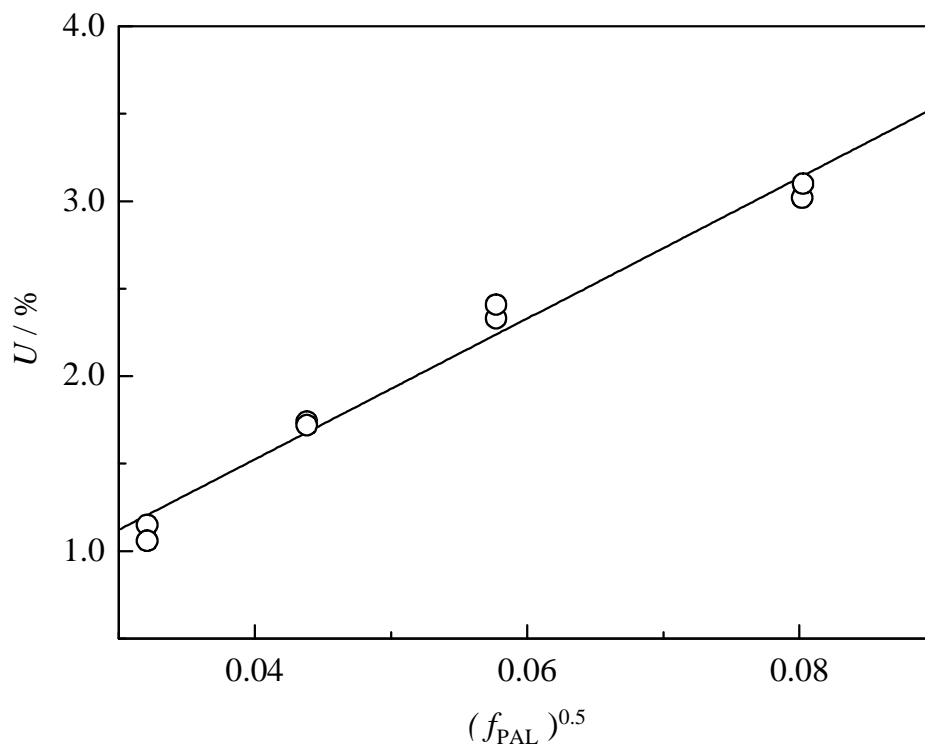
Abb. 6.1: Einfluß der Propionaldehydkonzentration auf den thermischen Grundumsatz in einer Ethen-Homopolymerisation ( p = 2000 \text{ bar} ; \tau_{\text{vWZ}} = 140 \text{ s} ; T = 260^\circ\text{C} )
