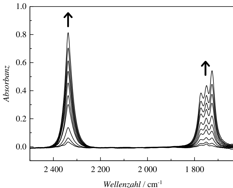
Abb. 5.2: Absorbanzspektrenserie während der thermischen Zersetzung von Tx-301 in n-Heptan bei 500 bar und 170°C (O=C=O Streckschwingung, C=O Streckschwingung)
