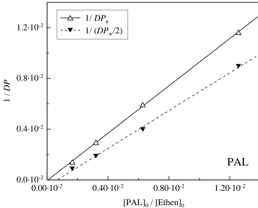
Abb. 4.3: Mayo-Auftragung für Ethen-Homopolymerisationen mit Propionaldehyd als Kettenüberträger ( p = 2000 \text{ bar} ; \tau_{\text{vWZ}} = 140 \text{ s} ; T_{\text{Mantel}} = 200^\circ\text{C} )
