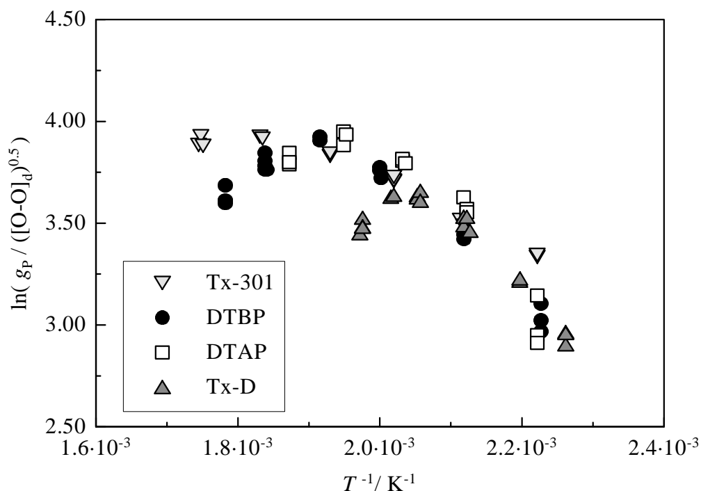
Abb. 6.18: Arrheniusdarstellung des reduzierten Umsatzes der in dieser Arbeit untersuchten Dialkylperoxide ( f_{\text{PAL}} = 3.3 \cdot 10^{-3} , m_E = 706 \text{ g}\cdot\text{h}^{-1} )
