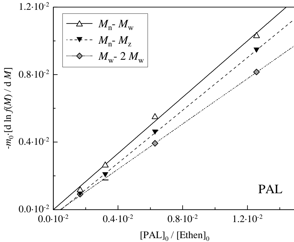
Abb. 4.9: CLD-Auftragung für die Ethen-Homopolymerisation mit Propionaldehyd als Kettenüberträger ( p = 2000 \text{ bar} ; \tau_{vWZ} = 140 \text{ s} ; T_{Mantel} = 200^\circ\text{C} )
