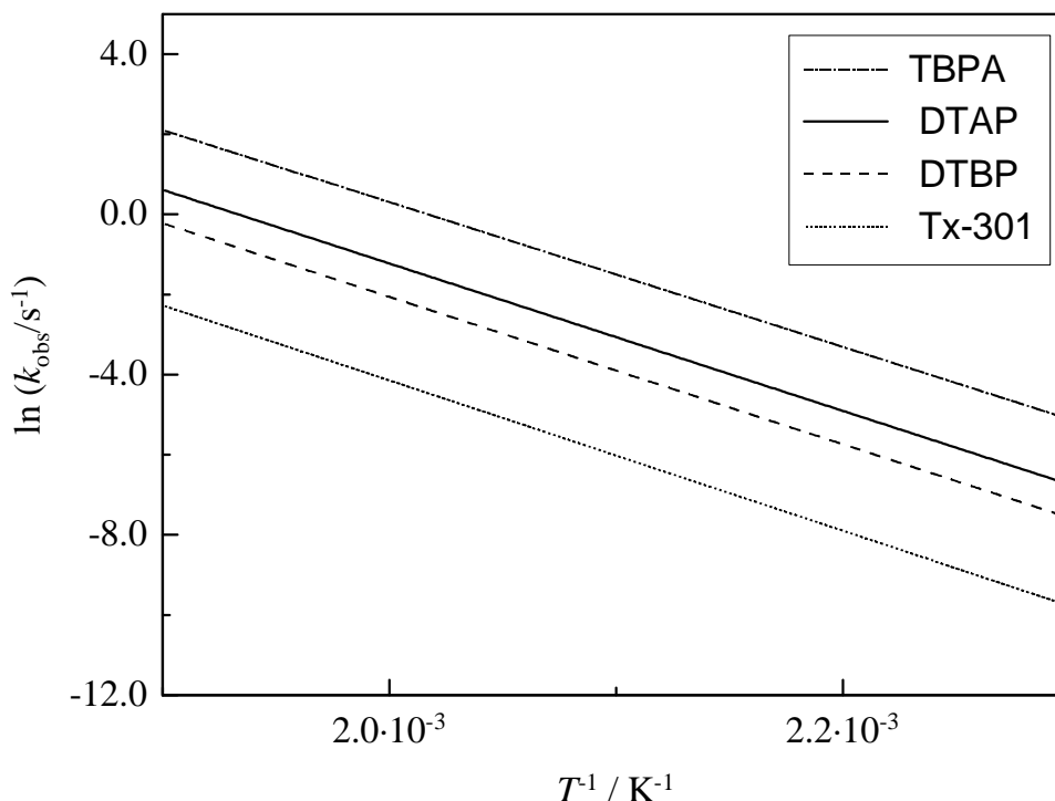
Abb. 5.8: Arrheniusauftragung für den Zerfall verschiedener Dialkylperoxide bei 2000 bar in n-Heptan
