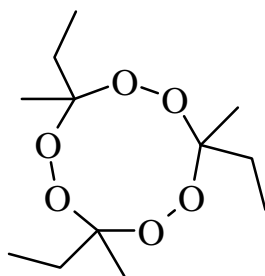
Abb. 5.1: Struktur des untersuchten 3,6,9-Triethyl-3,6,9-trimethyl-1,4,7-triperoxyanonans
