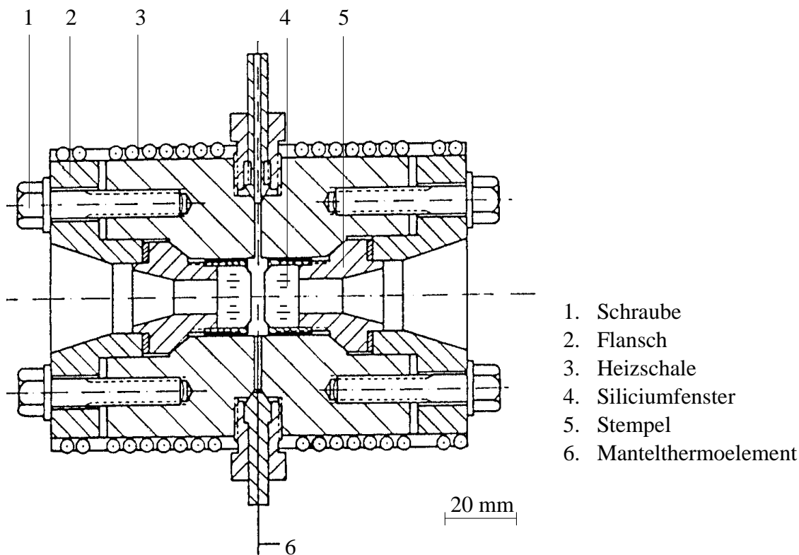
Abb. 3.1: Optische Hochdruckzelle
