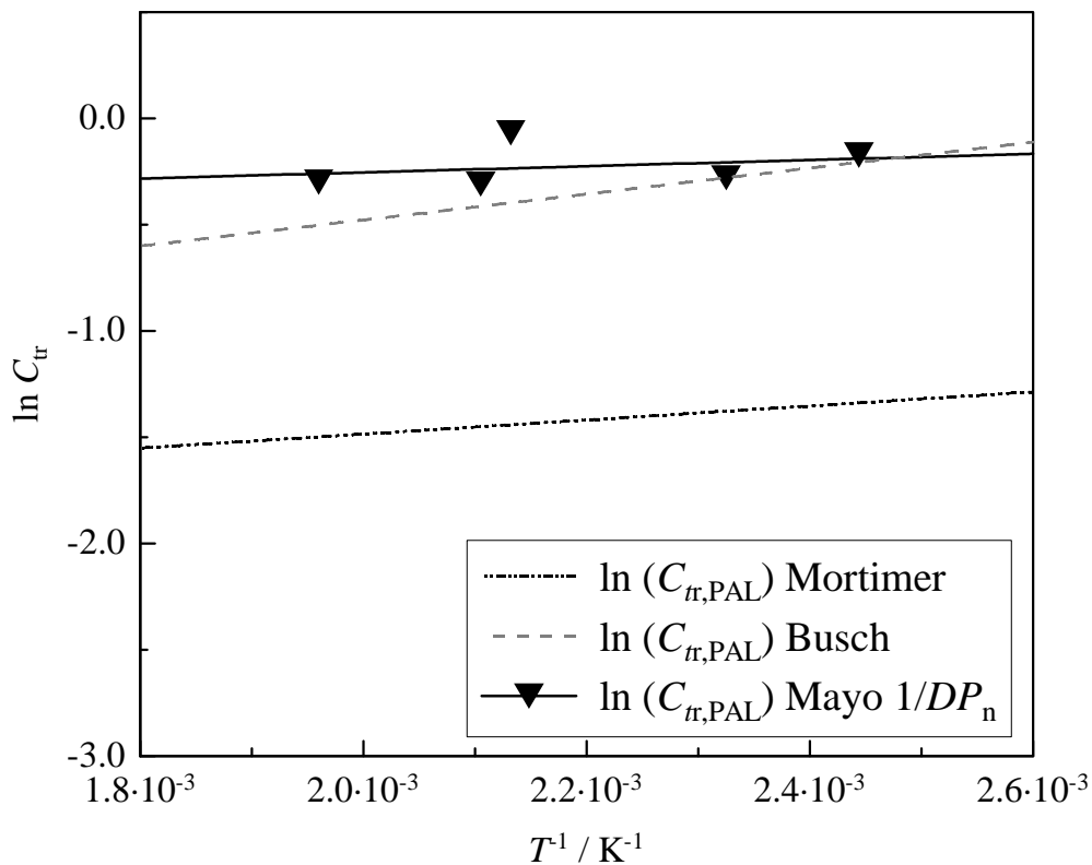
Abb. 4.13: Vergleich der in der vorliegenden Arbeit bestimmten Temperaturabhängigkeit der Transferkonstante von Propionaldehyd bei 2000 bar mit Daten von Mortimer [6] und Busch [3]
