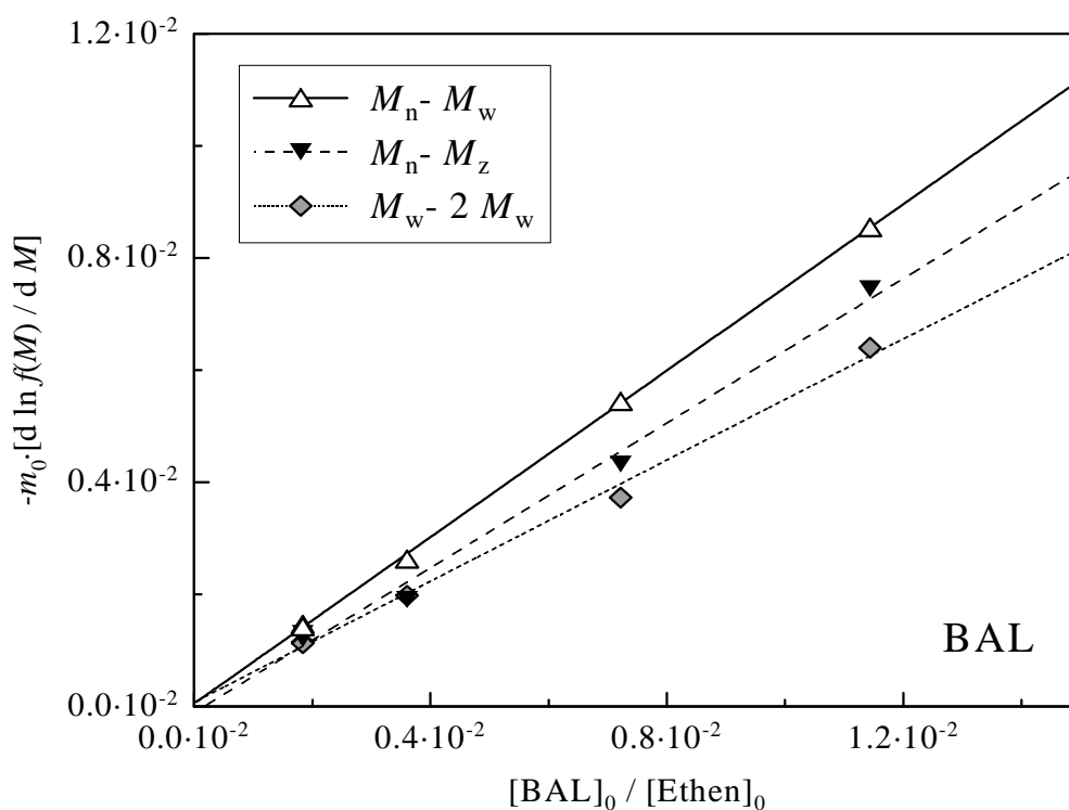
Abb. 4.8: CLD-Auftragung für die Ethen-Homopolymerisation mit Butyraldehyd als Kettenüberträger ( p = 2000 \text{ bar} ; \tau_{vWZ} = 140 \text{ s} ; T_{Mantel} = 200^\circ\text{C} )
