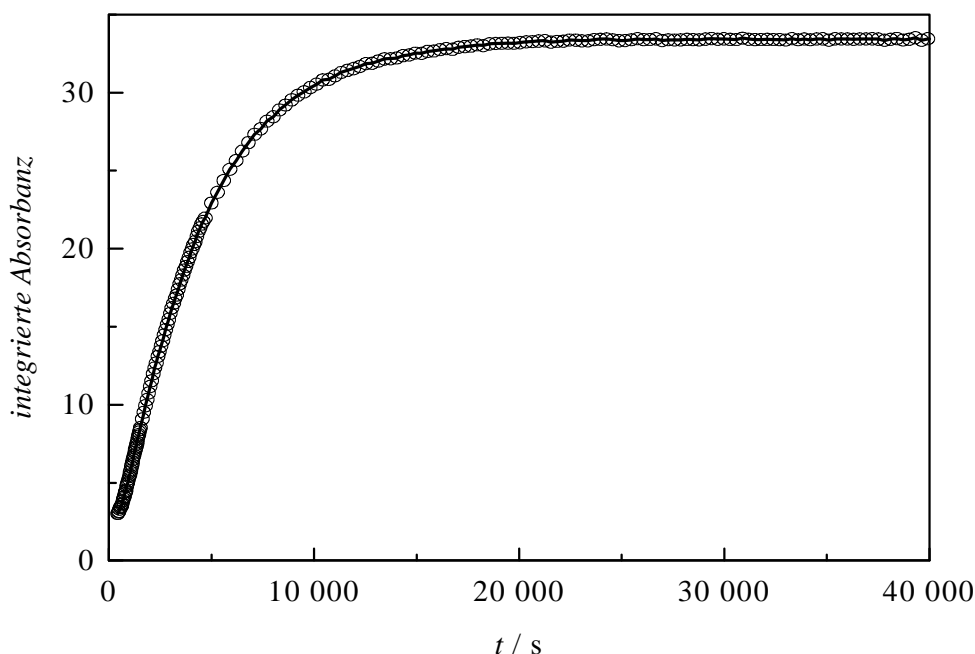
Abb. 5.5: Integrierte Absorbanz der Carbonylbande von 1690\text{ cm}^{-1} bis 1812\text{ cm}^{-1} (offene Kreise) als Funktion der Zeit für die thermische Zersetzung von Tx-301 in n-Heptan bei 500 bar und 170^\circ\text{C} ; die durchgezogene Linie wird durch nicht-lineare Regression nach Gleichung 5.1 erhalten
