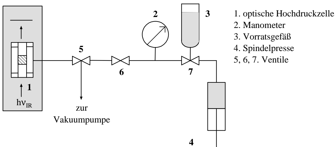
Abb.3.2: Schematischer Aufbau des Druckzweiges für die Satzreakorteknik.
