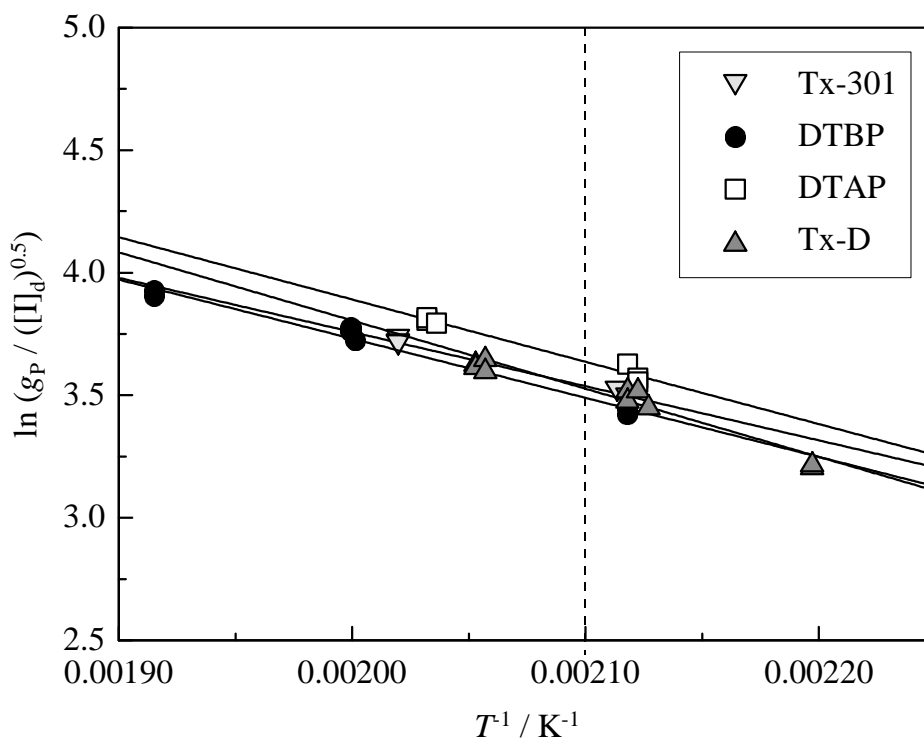
Abb. 6.20: Arrheniusdarstellung des reduzierten Umsatzes der in dieser Arbeit untersuchten Dialkylperoxide für Temperaturen unterhalb von T_{\text{opt}} und im Umsatzbereich von 4 % bis 8 % ( f_{\text{PAL}} = 3.3 \times 10^{-3} , m_E = 706 \text{ g h}^{-1} )
