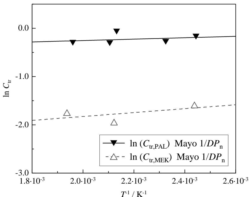
Abb. 4.14: Vergleich der in der vorliegenden Arbeit bestimmten Temperaturabhängigkeit der Transferkonstante von Propionaldehyd und Methylethylketon bei 2000 bar
