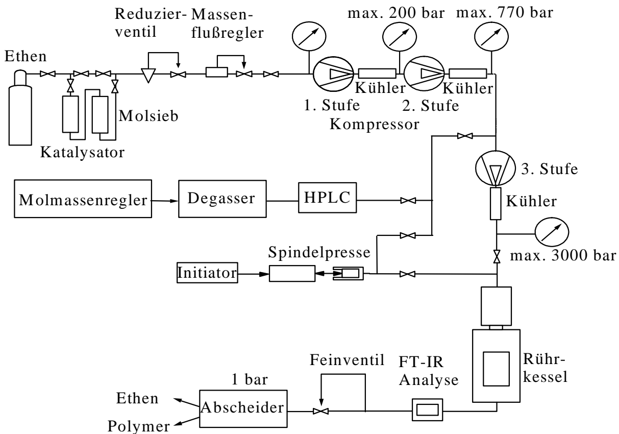
Abb. 3.3: Schematische Darstellung der Mini-Technikumsanlage.
