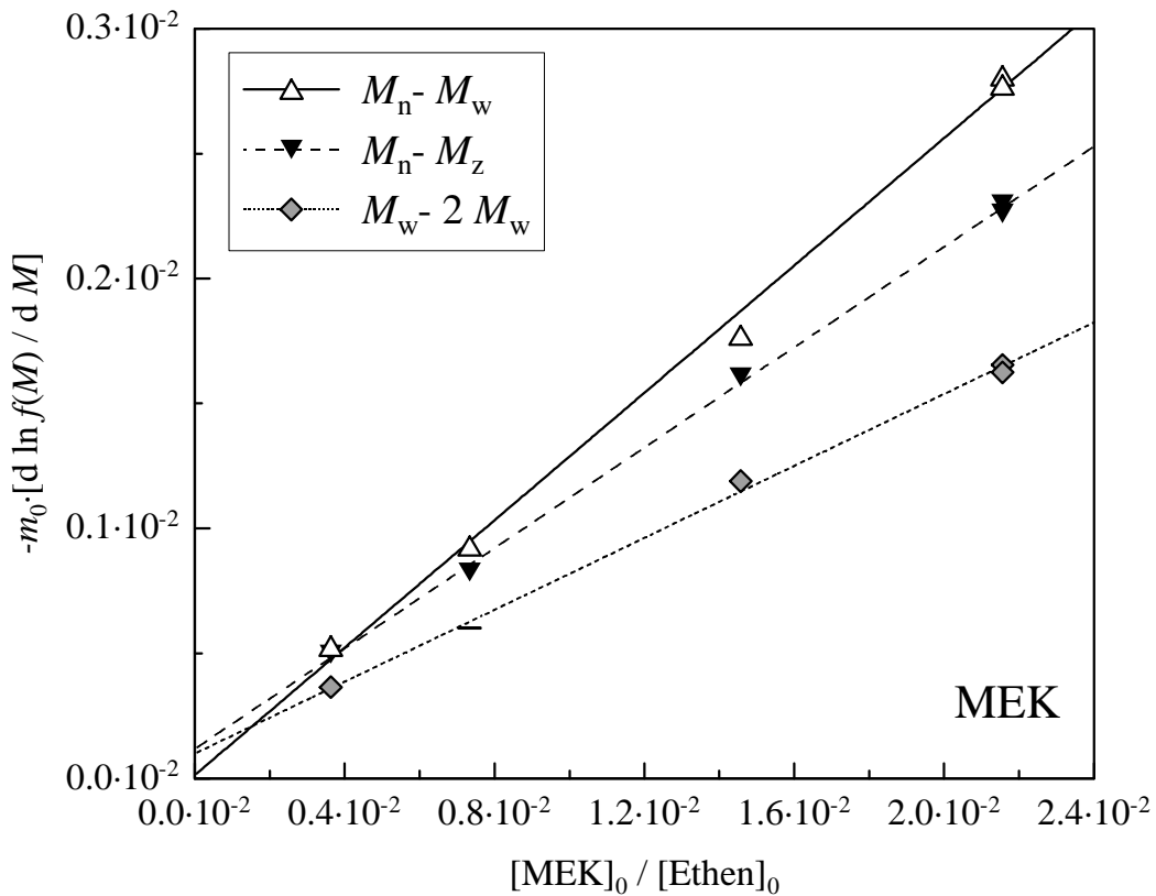
Abb. 4.10: CLD-Auftragung für die Ethen-Homopolymerisation mit Methyl ethyl keton als Kettenüberträger ( p = 2000 \text{ bar} ; \tau_{vWZ} = 140 \text{ s} ; T_{Mantel} = 200^\circ\text{C} )
