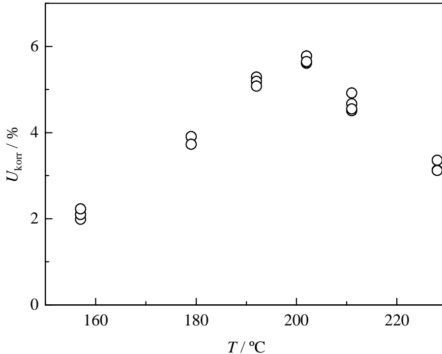
Abb. 6.5: Korrigiertes Umsatz-Temperatur-Profil für das in Abbildung 6.4 dargestellte Experiment
