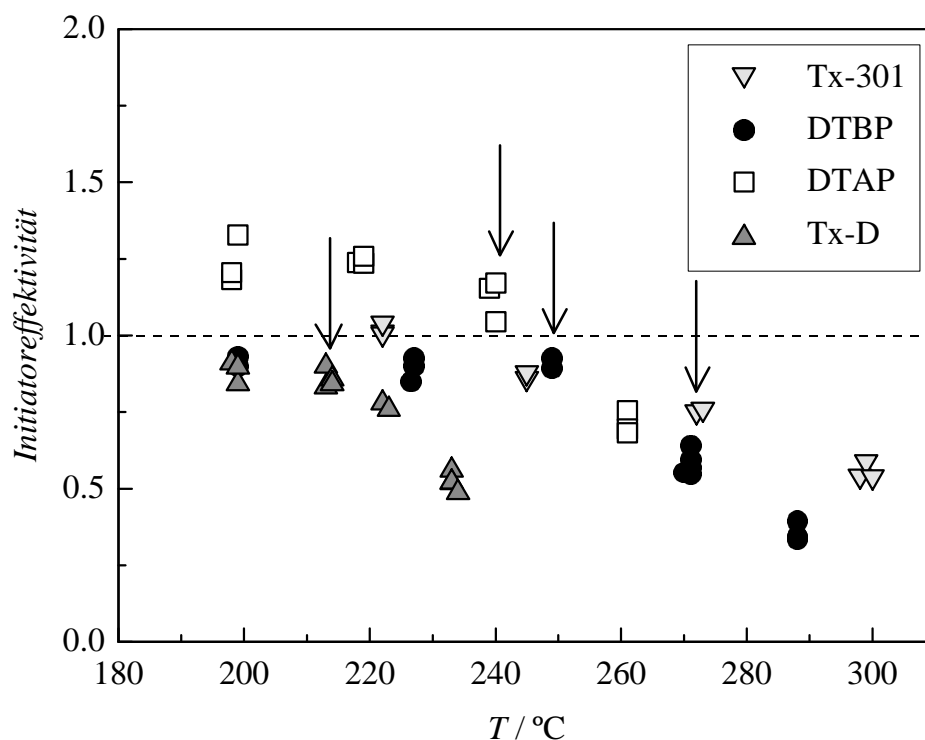
Abb. 6.22: Temperaturabhängigkeit der Initiatoreffektivität (Methode 1) der in dieser Arbeit untersuchten Dialkylperoxide ( f_{PAL} = 3.3 \times 10^{-3} , m_E = 706 \text{ g}\cdot\text{h}^{-1} )
