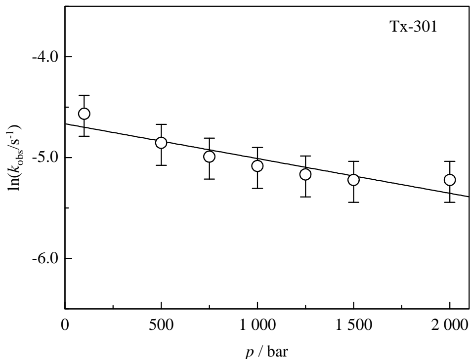
Abb. 5.7: Druckabhängigkeit der Zerfallsgeschwindigkeitskoeffizienten von Tx-301 bei 210°C in n -Heptan
