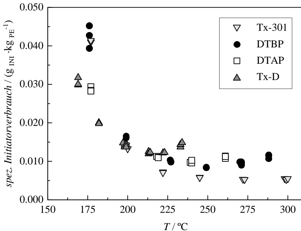
Abb. 6.28: Temperaturabhängigkeit des spezifischen Initiatorverbrauchs der in dieser Arbeit untersuchten Dialkylperoxide ( f_{PAL} = 3.3 \cdot 10^{-3} , m_E = 706 \text{ g h}^{-1} )
