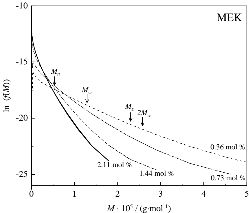
Abb. 4.7: Einfluß der Methylethylketonkonzentration auf die Zahlenverteilung des Molekulargewichts von Polyethylen ( p = 2000 \text{ bar} ; \tau_{\text{vWZ}} = 140 \text{ s} ; T_{\text{Mantel}} = 200^\circ\text{C} )
