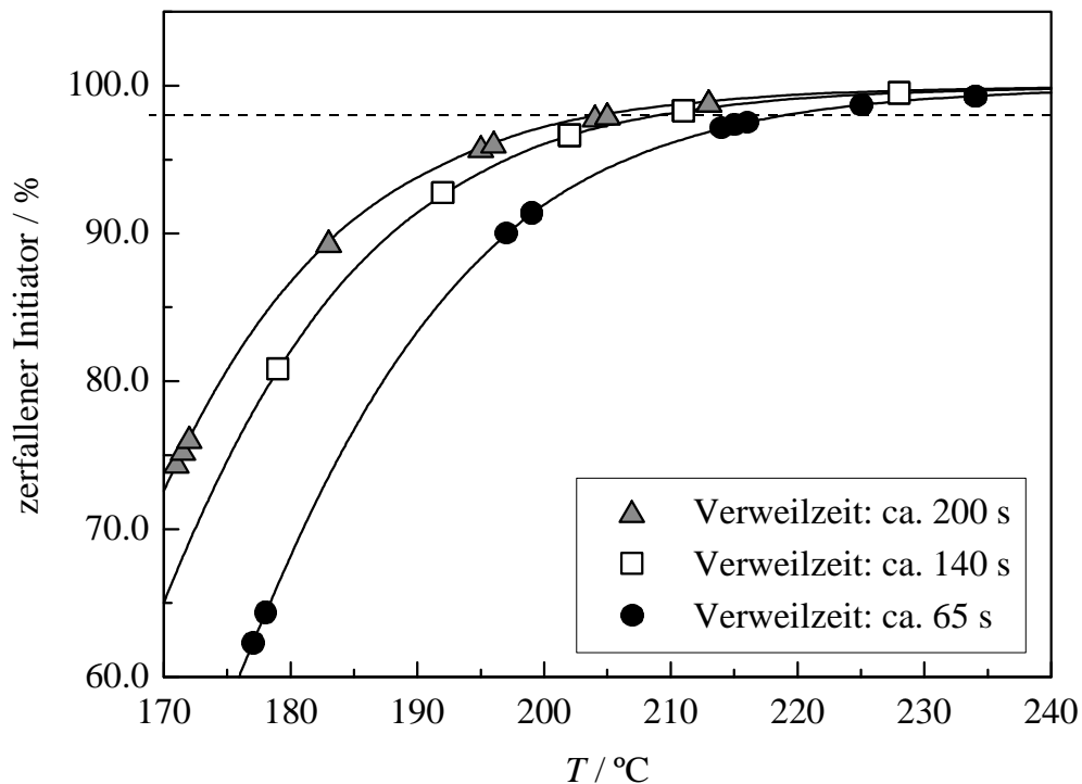
Abb. 6.12: Einfluß der Verweilzeit auf die Temperaturabhängigkeit des Initiatorumsatzes von TBPA im idealen Rührkessel ( p = 2000 \text{ bar} )
