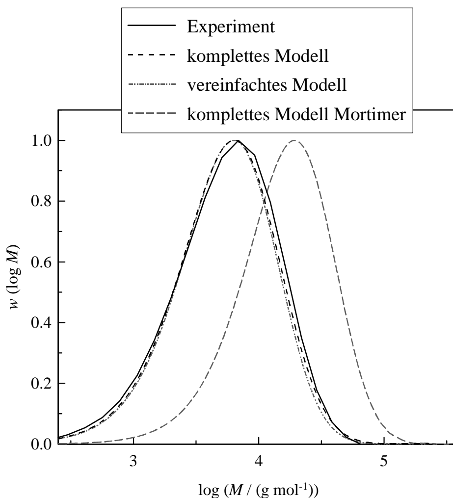
Abb. 4.11: Vergleich von experimenteller und modellierten Molekulargewichtsverteilungen für die Ethen-Homopolymerisation mit 1.13 mol % BAL als Kettenüberträger ( p = 2000 \text{ bar} ; \tau_{VWZ} = 140 \text{ s} ; T_{\text{Mantel}} = 200^\circ\text{C} )
