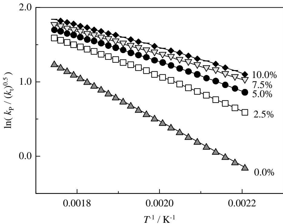
Abb. 6.19: Arrheniusdarstellung von k_p / (k_t)^{0.5} für verschiedene Monomerumsätze von 0 bis 10 % ( p = 2000 \text{ bar} )
