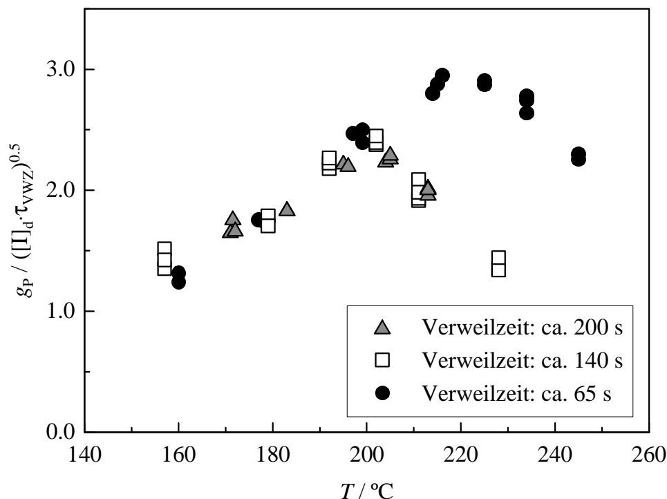
Abb. 6.11: Verweilzeitunabhängiger reduzierter Monomerumsatz für die in Abb. 6.10 gezeigten Meßreihen
