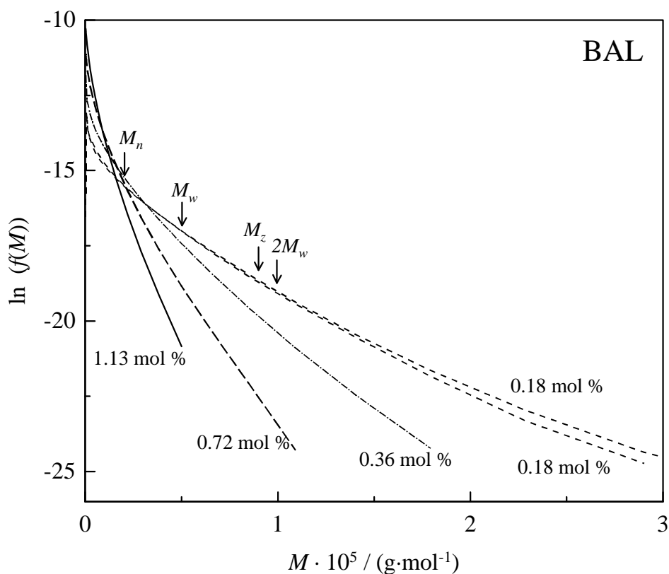
Abb. 4.5: Einfluß der Butyraldehydkonzentration auf die Zahlenverteilung des Molekulargewichts von Polyethylen ( p = 2000 \text{ bar} ; \tau_{VWZ} = 140 \text{ s} ; T_{\text{Mantel}} = 200^\circ\text{C} )
