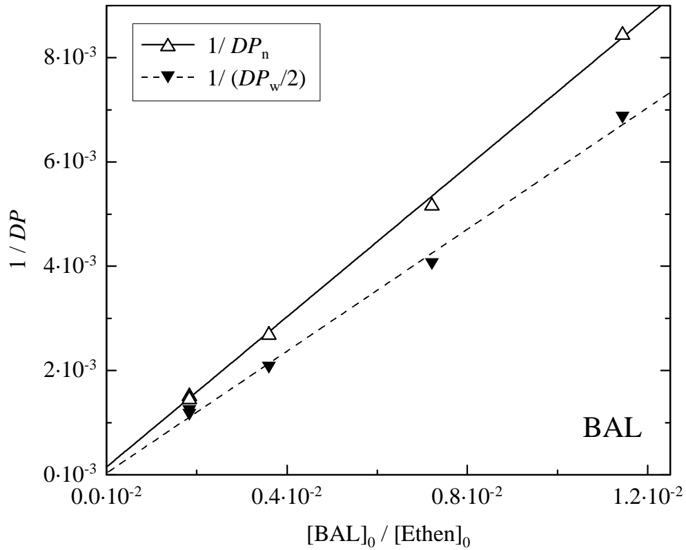
Abb. 4.2: Mayo-Auftragung für Ethen-Homopolymerisationen mit Butyraldehyd als Kettenüberträger ( p = 2000 \text{ bar} ; \tau_{\text{vWZ}} = 140 \text{ s} ; T_{\text{Mantel}} = 200^\circ\text{C} )
