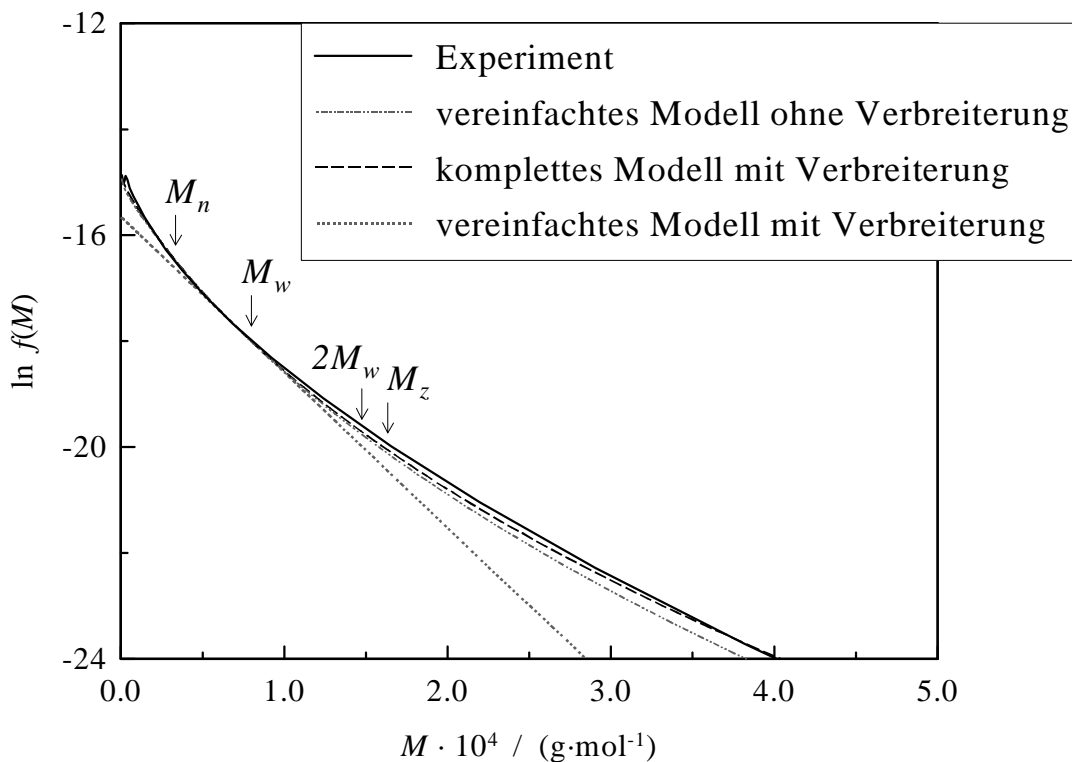
Abb. 4.12: Vergleich von experimenteller und modellierter Zahlenverteilungen in der Ethen-Homopolymerisation mit 1.13 mol % BAL als Kettenüberträger ( p = 2000 \text{ bar} ; \tau_{\text{VWZ}} = 140 \text{ s} ; T_{\text{Mantel}} = 200^\circ\text{C} )
